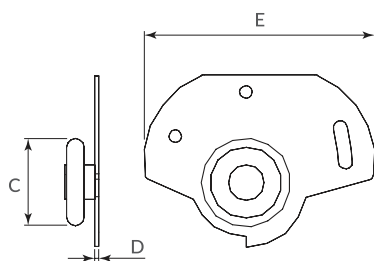
Rodadura inferior (incluye 4 piezas)
